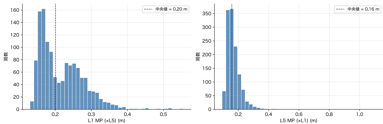
図 7: マルチパス RMS 分布 — L1/L5 ペア(MP15 = L5 をパートナーとする L1 マルチパス、MP51 = L1 をパートナーとする L5 マルチパス)。コアベースライン。
