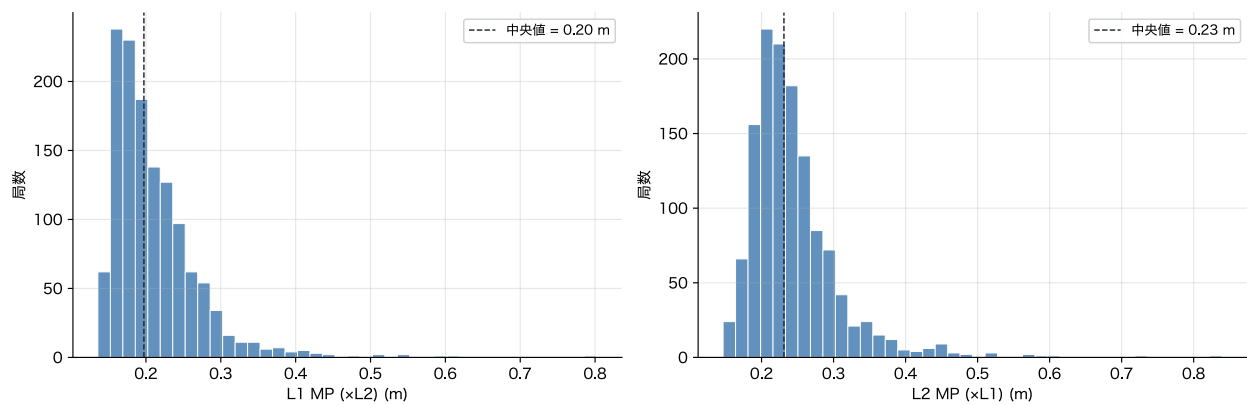
図 6: マルチパス RMS 分布 — L1/L2 ペア(MP12 = L2 をパートナーとする L1 マルチパス、MP21 = L1 をパートナーとする L2 マルチパス)。Shiono & Kubo 2025 のコアベースライン。
