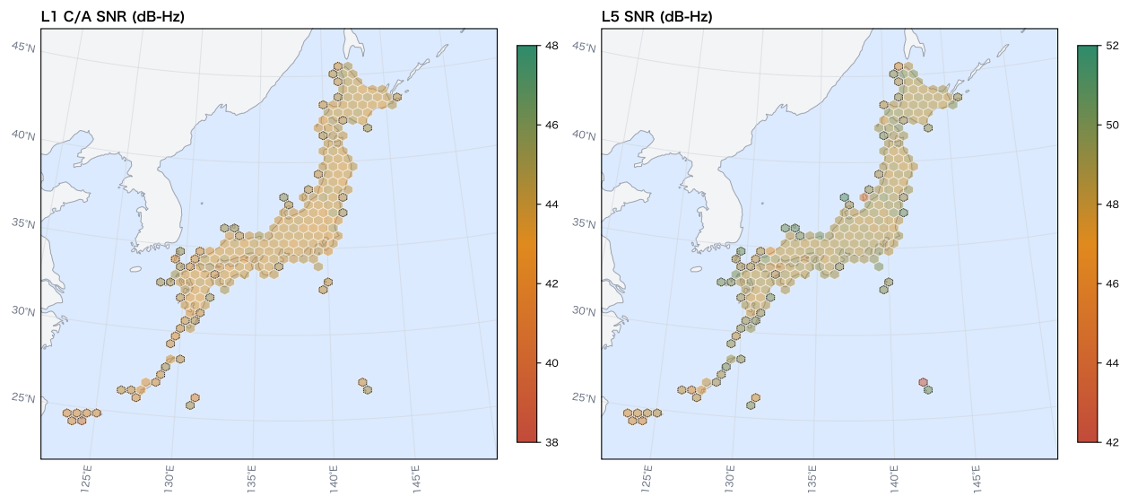
図 10: 基準局・月間の SNR — L1 C/A と L5(コアベースライン)。信号ごとに固有のカラーズケール。
