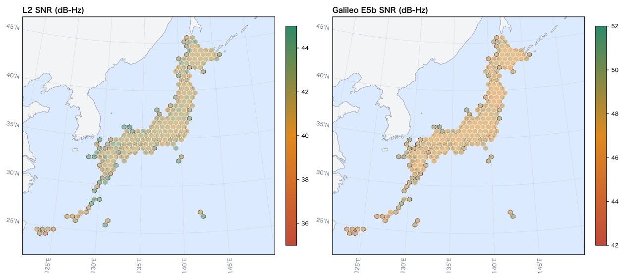
図 11: 基準局・月間の SNR — L2(コア)と Galileo E5b(参考。絶対評価ベースラインには含まれない)。信号ごとに固有のカラーズケール。
