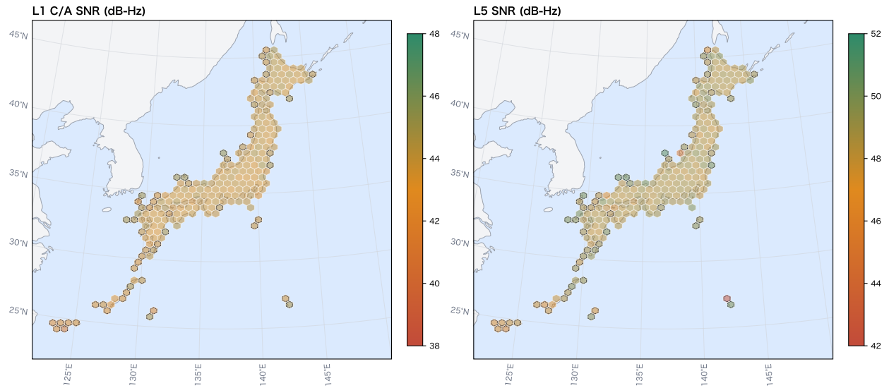
図 10: 基準局・月間の SNR — L1 C/A と L5(コアベースライン)。信号ごとに固有のカラーズケール。
